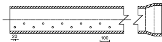
Corte longitudinal
